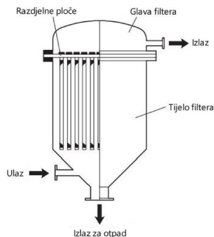
Slika 2.8. Candle filter [1].
