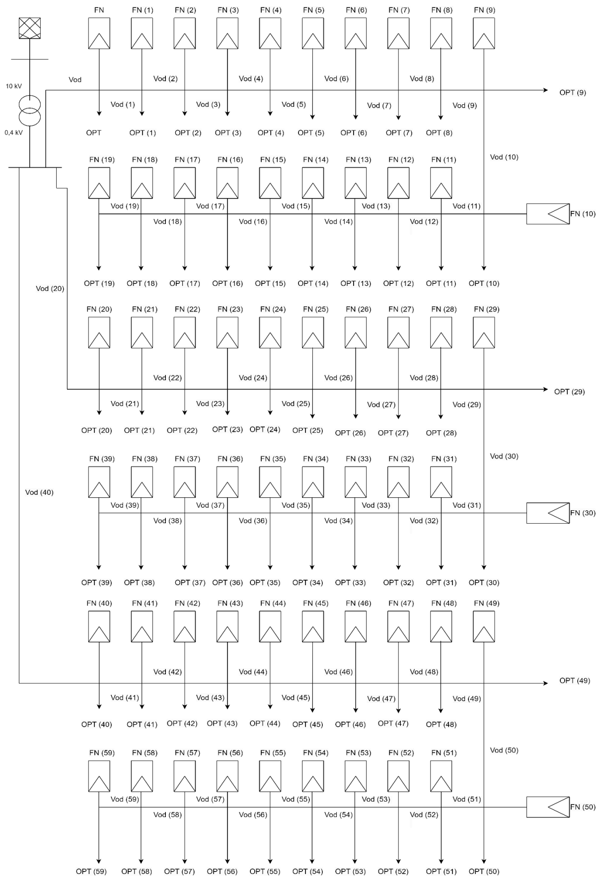
Slika 4.2. – Testna niskonaponska mreža Špansko
