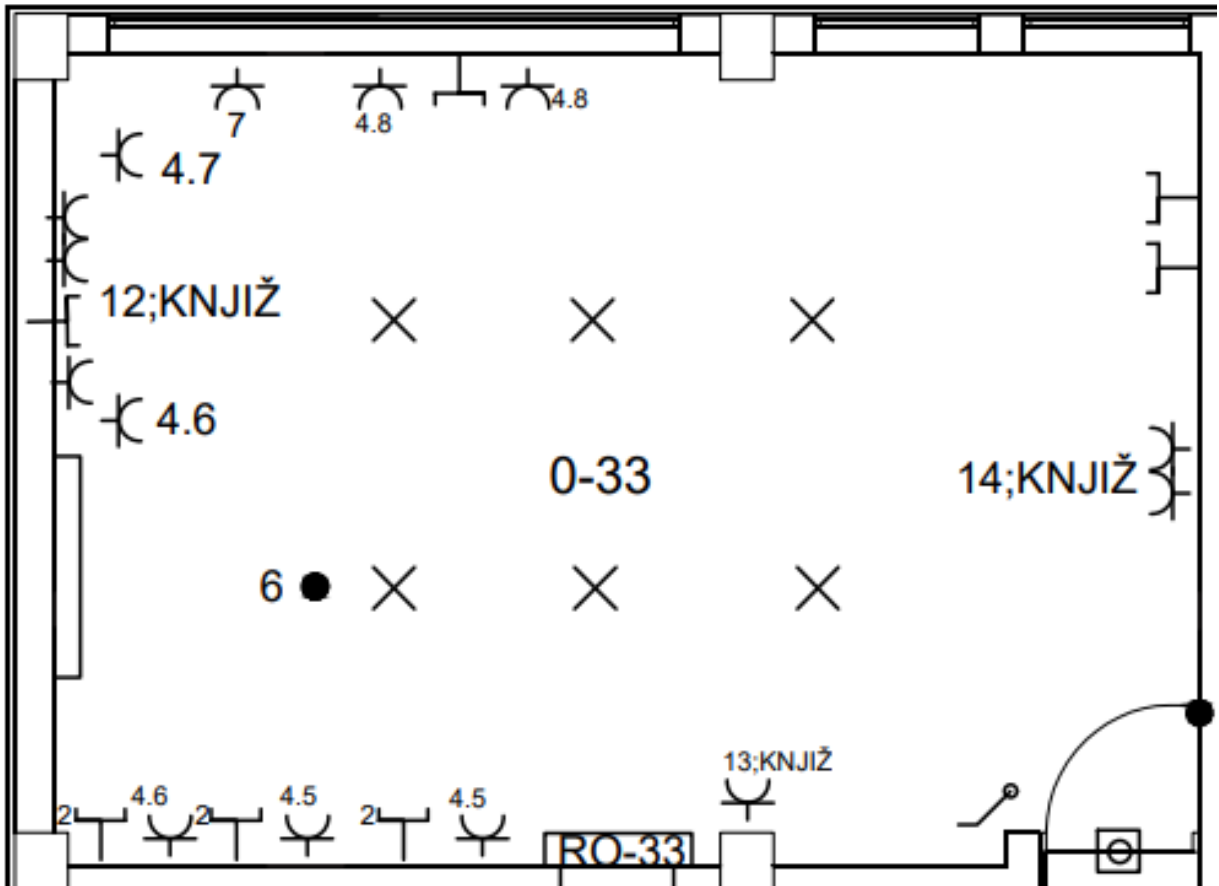
Slika 4.7. Tlocrt predavaonice 0-33
