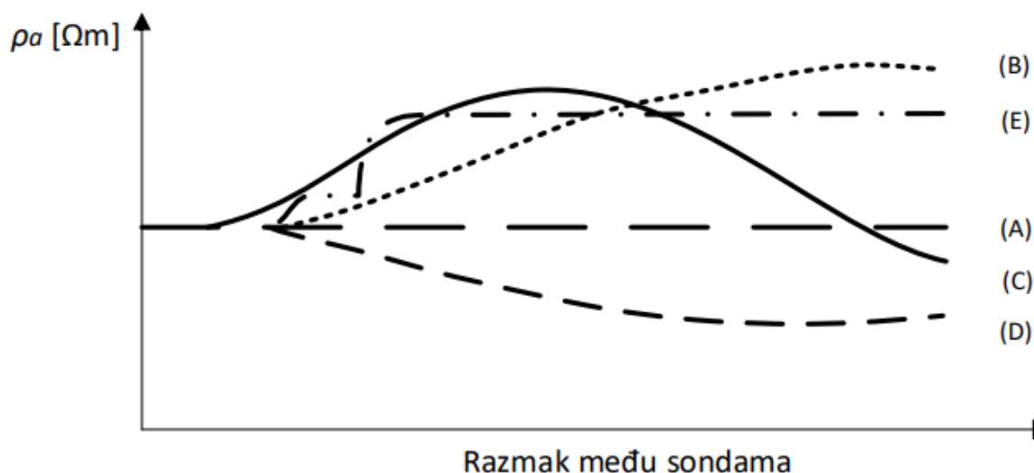
Slika 3.1. Tipične krivulje prividnog specifičnog otpora tla [5]
