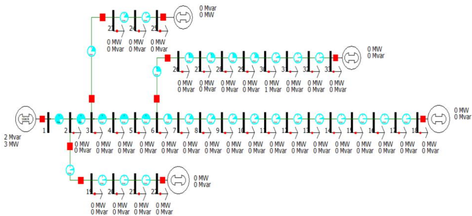
Slika 5.1. Prikaz 33 sabirničke testne mreže
