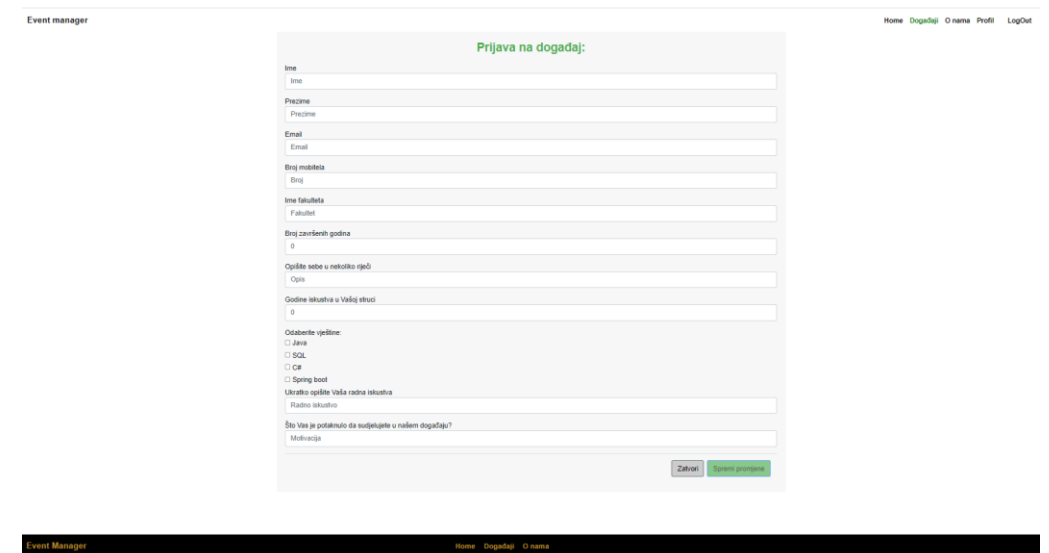
Slika 5.8. Komponenta EventComponent
