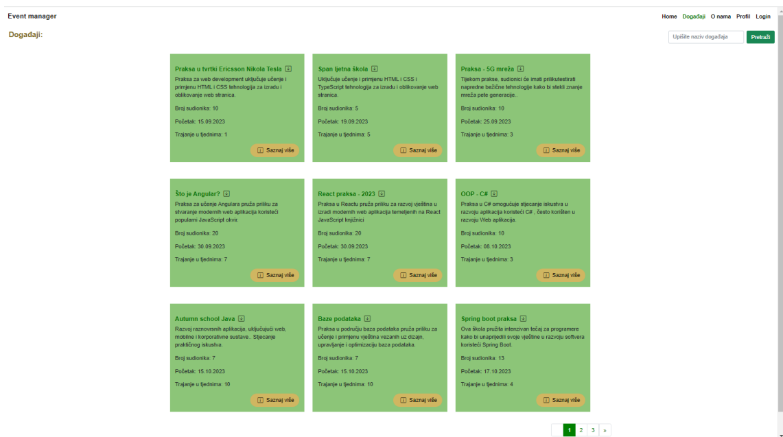
Slika 5.5. Komponenta EventsComponent
