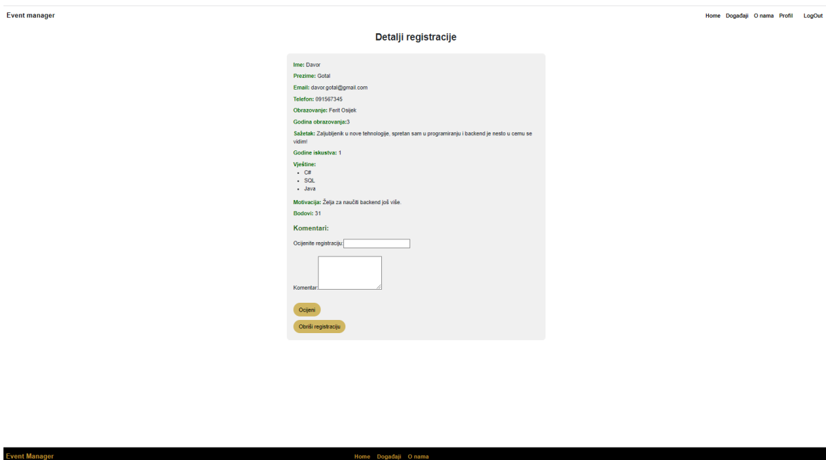
Slika 5.21. RegistrationDetailsComponent komponenta
