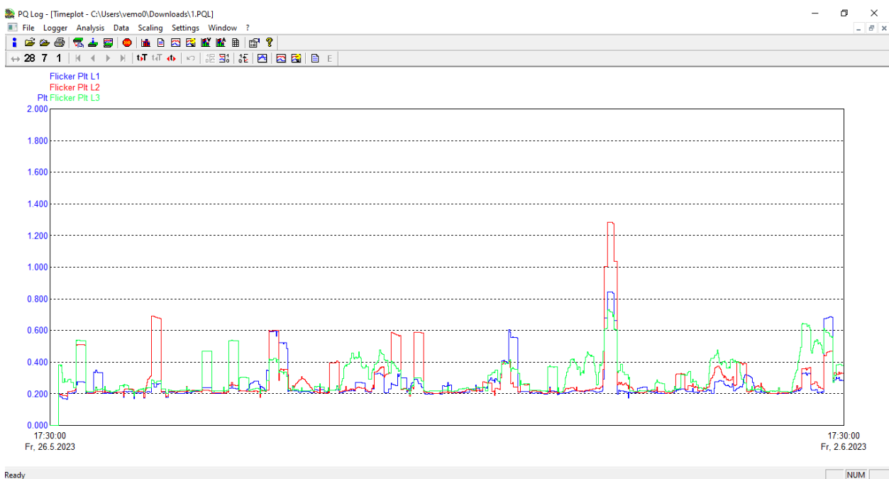
Slika 4.8. Prikaz treptaja napona (flickeri)
