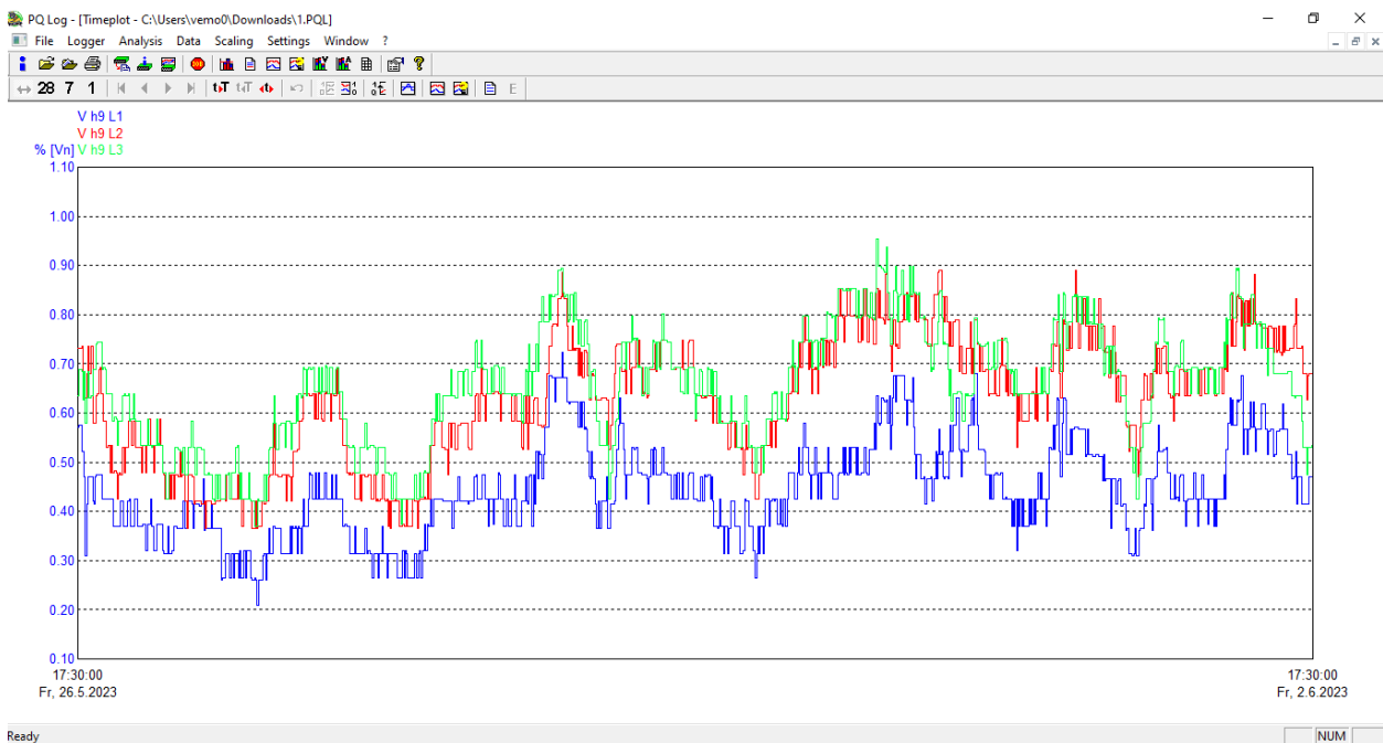
Slika 4.14. Napon 9. harmonika
