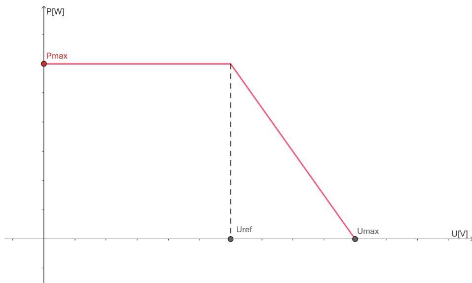
Slika 3.3. Volt/Watt krivulja [7]
