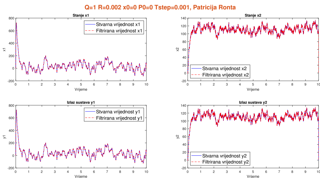
Slika 5.48: Rad Kalman filtra kada je \mathbf{Q} = 1
