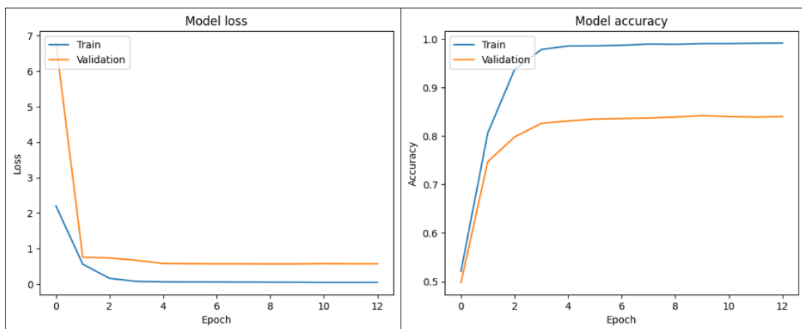
Slika 4.17. Validacijski gubitak i gubitka na treniranju te točnost na validacijskom skupu i točnost na skupu za treniranje – model s ResNet101 arhitekturom kao ekstraktorom značajki
