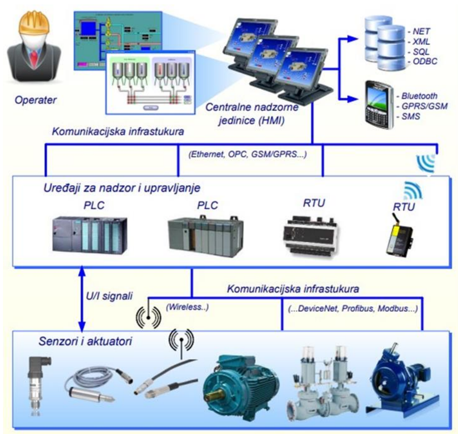
Slika 2.1. Kompletna infrastruktura sustava za nadzor i upravljanje [6]
