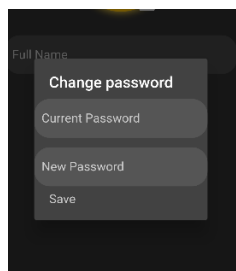
Slika 5.11 Promjena lozinke
