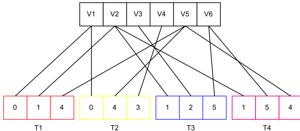
Slika 3.3 Prikaz vertex i index buffera te njihovih odnosa
