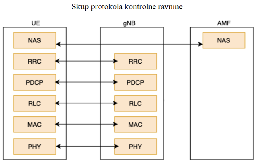
Slika 3.4. 5G skup protokola kontrolne ravnine [13]
