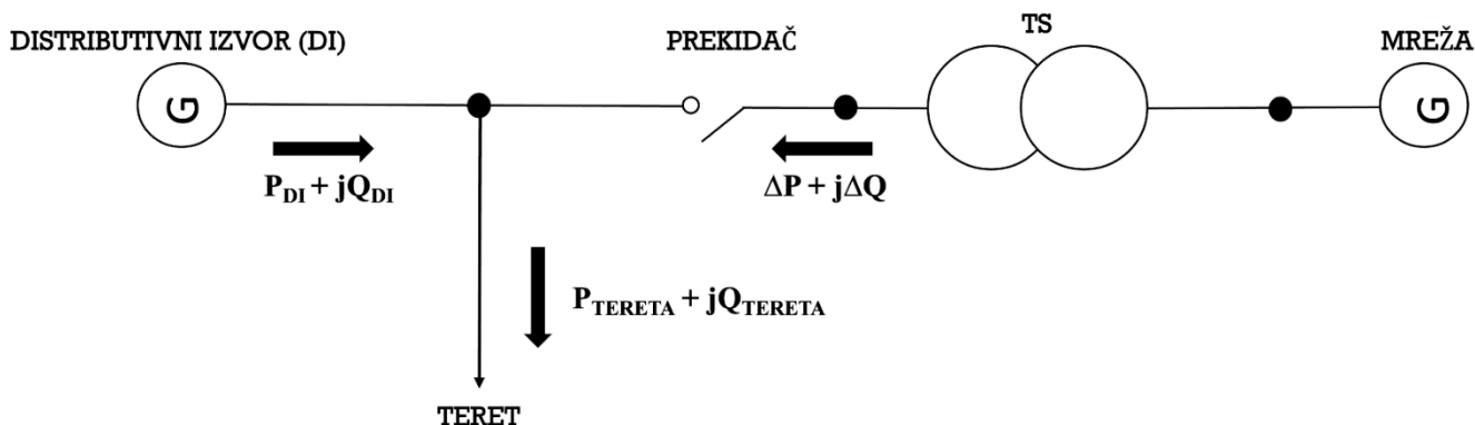
Slika 3.1. Prikaz tokova snaga između DI s mrežom za vrijeme otopnog pogona pomoću nadomjesne sheme [2]
