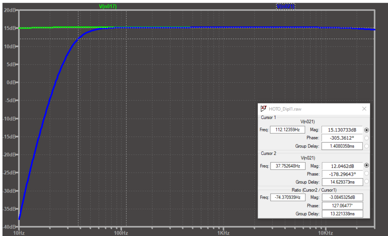
Slika 3.10. Amplitudno frekvencijska karakteristika visoko-propusnog filtera
