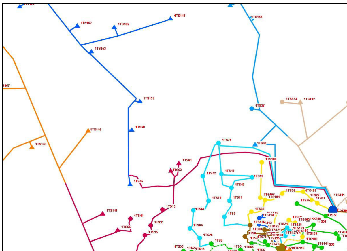
Slika 7-11 Početno stanje napajanja 10 kV DV Trnovac – DV PPK Požega zapad
