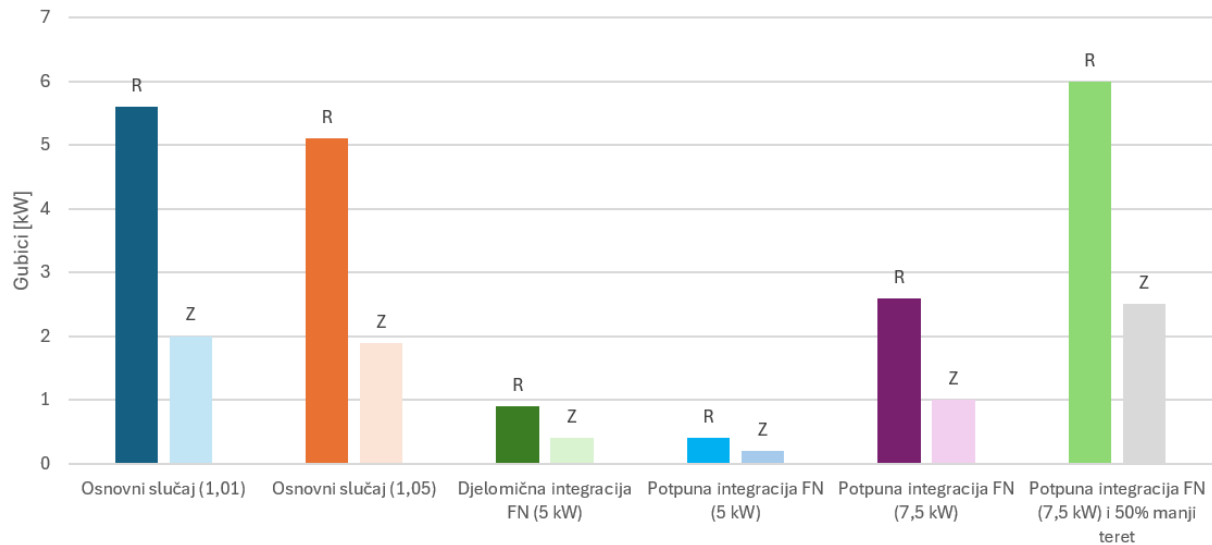
Slika 5.31. Usporedba gubitaka radikalne i zamkaste mreže za sve scenarije
