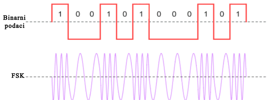
Slika 2.13: FSK modulacijski postupak [33]
