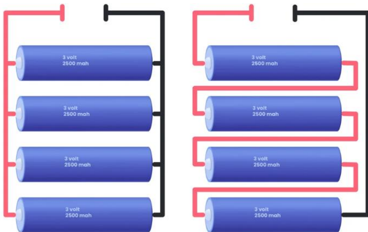
Slika 2.5. Paralelni spoj (lijevo) i serijski spoj (desno)
