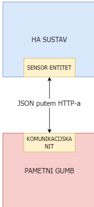
Slika 3.11. Arhitektura integracije
