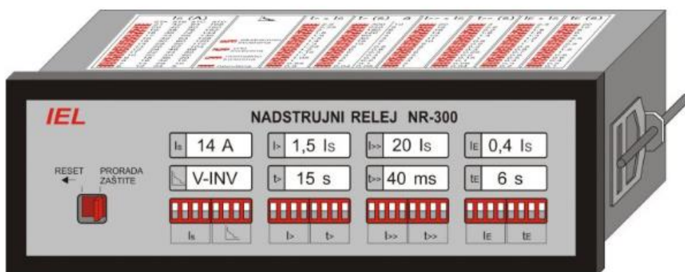
Slika 4.9. Nadstrujni relej [27]
