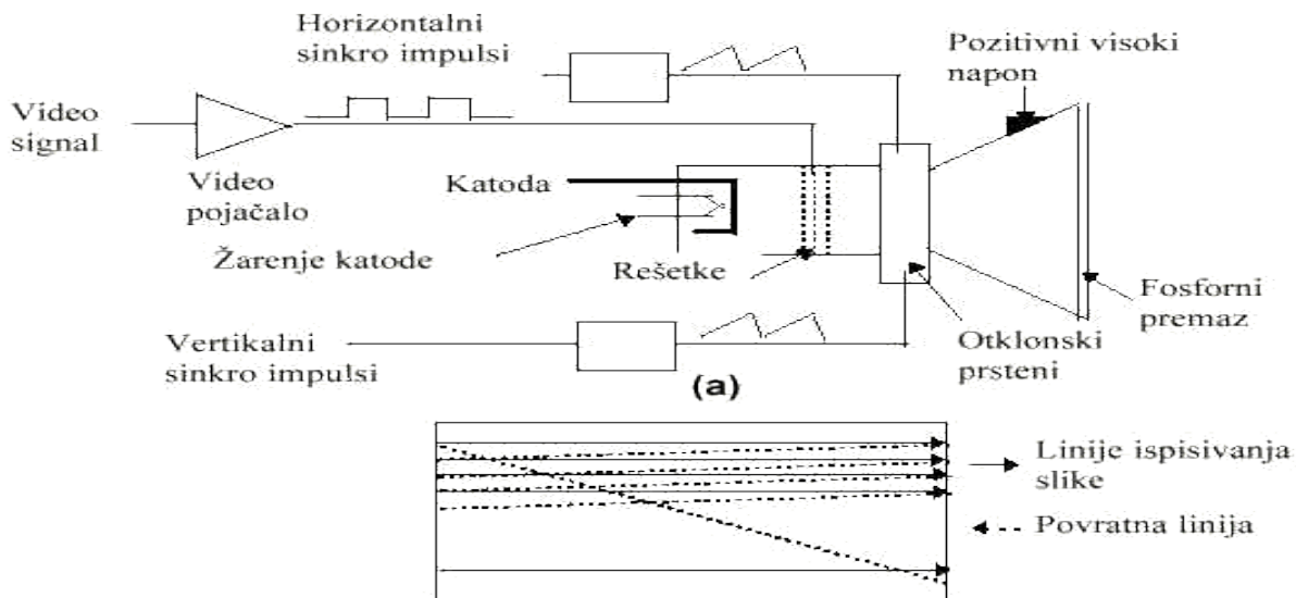
Slika 2.5. Katodna cijev [1]
