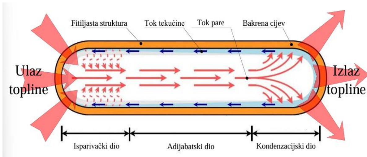
Slika 5.1. Građa toplinske cijevi
