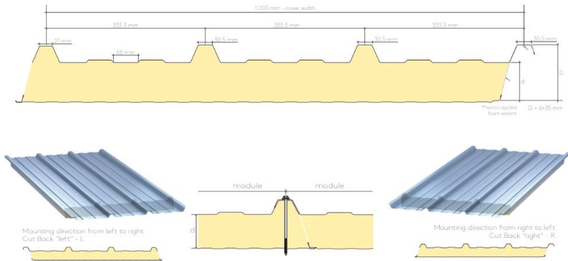
Slika 4.11. Dimenzije krovnog pokrivača [14]
