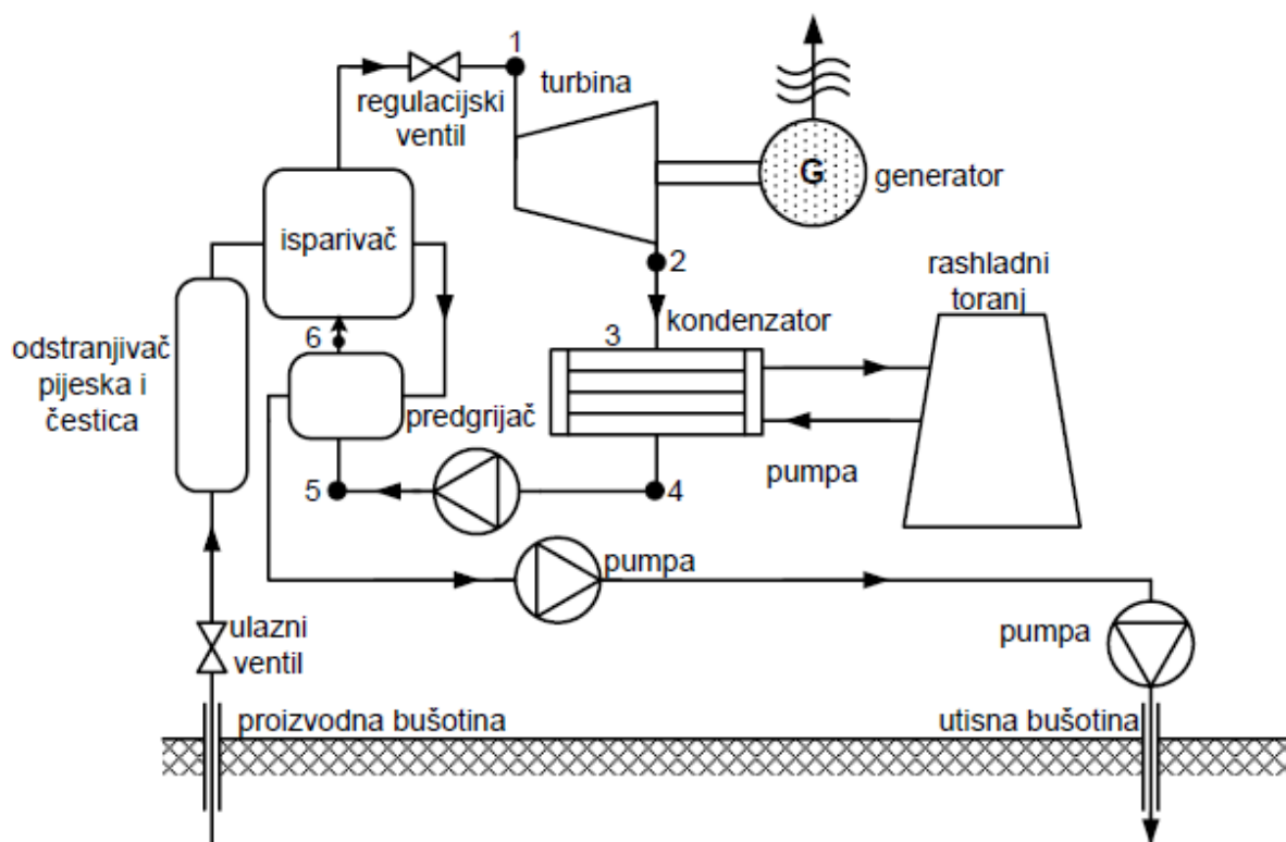
Slika 3.10. Geotermalna elektrana s binarnim ciklusom (ORC) [5]
