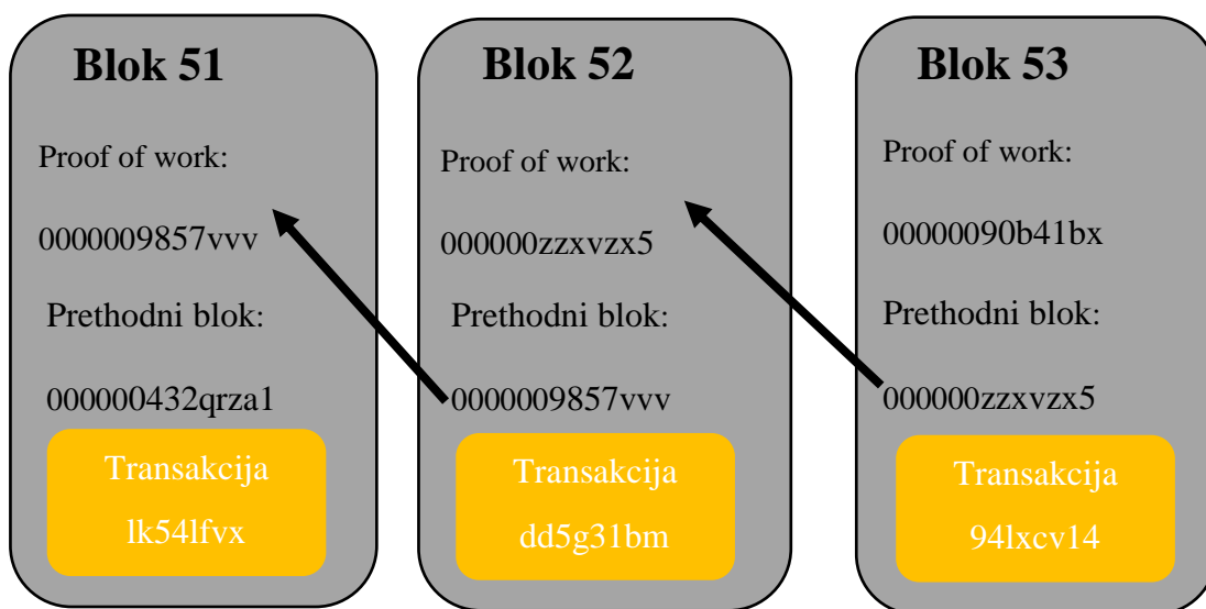
Slika 2. Prikaz jednog lanca blokova [3]
