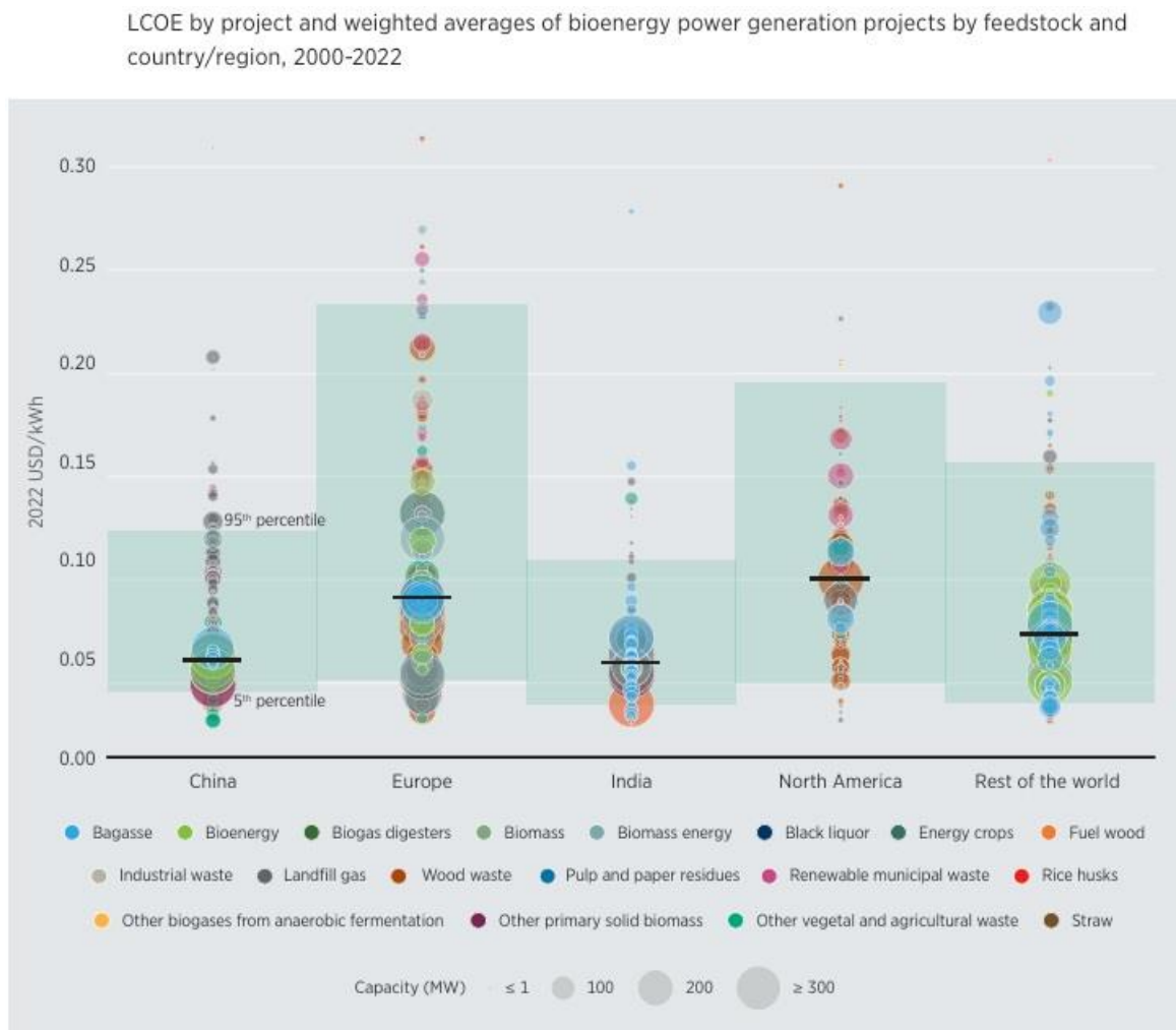
Slika 4.2. Rasponi LCOE-a i težinski prosjeci elektrana na biomasu po sirovinama i zemljama ili regijama u razdoblju od 2000. do 2022. godine [4]
