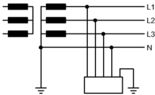
Slika 6.4. TT sustav, [10]
