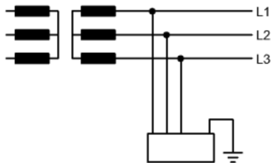
Slika 6.5. IT sustav, [10]
