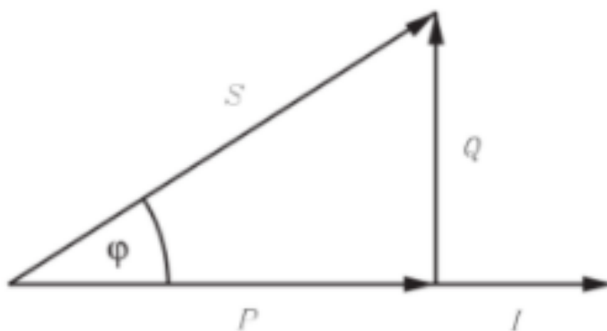
Slika 2.4. Trokut snage [2].
