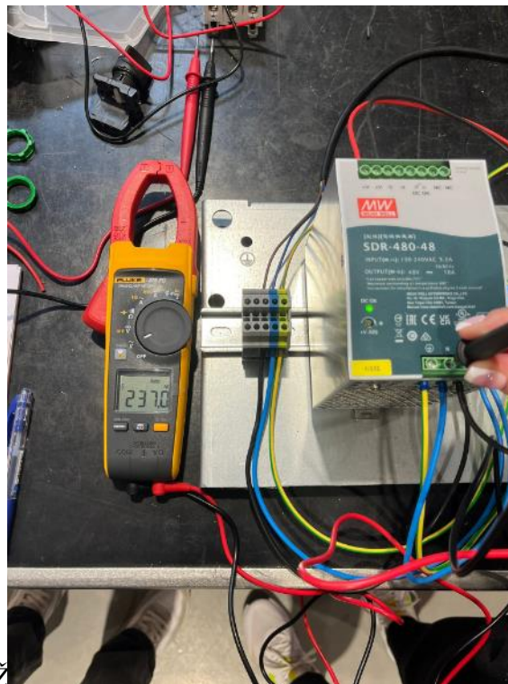
Slika 5.1.5. Mjerenje ulaznog napona s FLUKE 376 FC strujnim klještima
