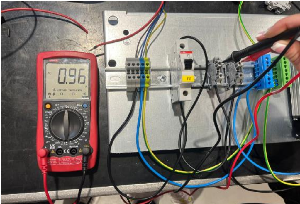
Slika 5.3.4. Mjerenje AC struje s UNI-T UT58C multimetrom
