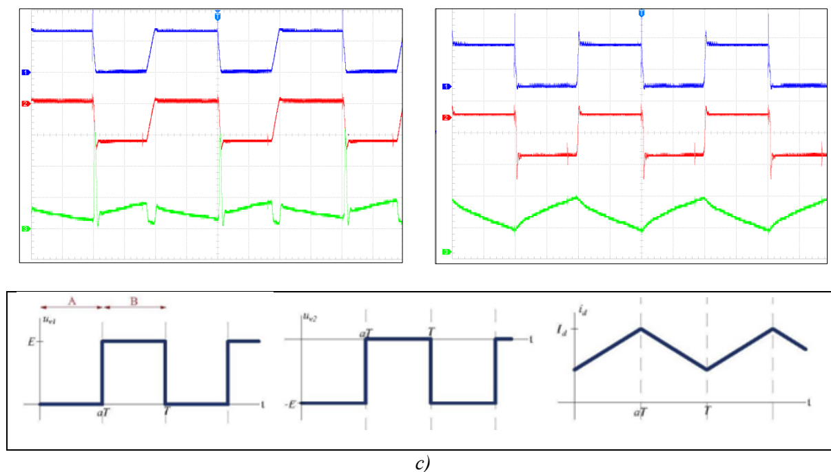
Slika 6.10. Uspoređivanje valnih oblika maketa i provedene analize za jednu odabranu radnu točku
