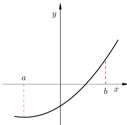
Slika 2.3. Funkcija s jednom nultočkom u intervalu [a,b] [2]
