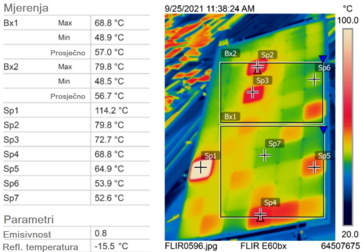
Sl. 3.9. Prikaz vrućih točaka na fotonaponskom modulu [12]
