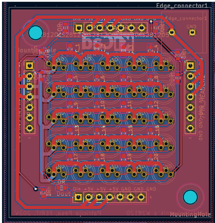
Sl. 3.4. Prikaz spojenih komponenta na tiskanoj pločici.
