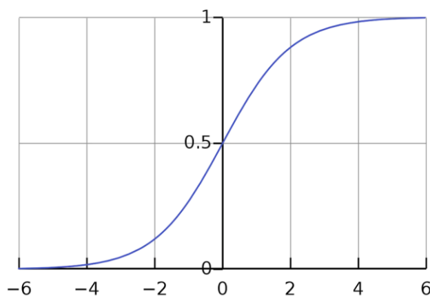
Slika 3.1. Sigmoid funkcija [11]
