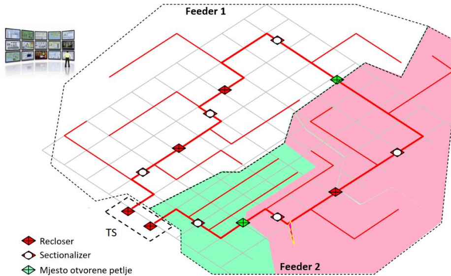
Slika 4-5 Trenutak kvara
