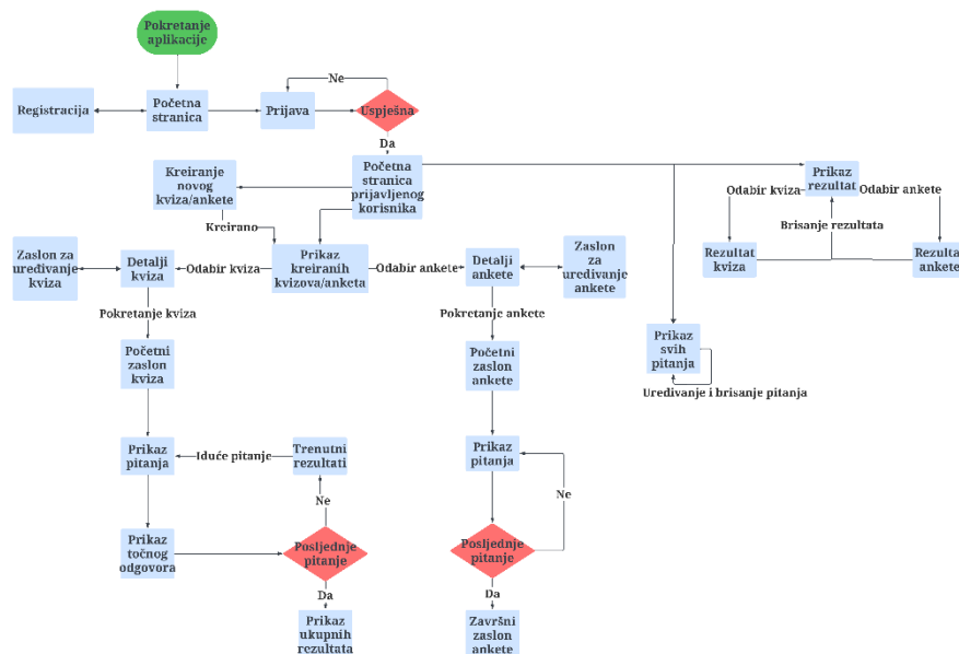
Slika 3.1. Dijagram toka za kreatora
