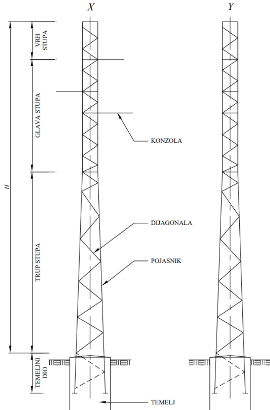
Slika 3.6. Konstrukcija čelično-rešetkastog stupa nadzemnog voda [13].
