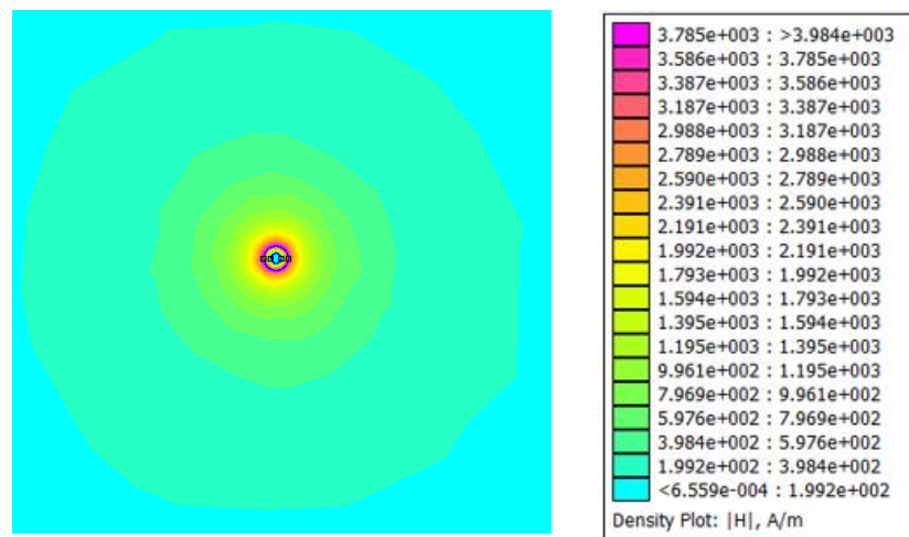
Slika 5.47. Prikaz jakosti magnetskog polja nadzemnog voda oblika glave stupa Jela u neposrednoj blizini vodiča s trenutnom vrijednosti struje i_3 = 97,81 A
