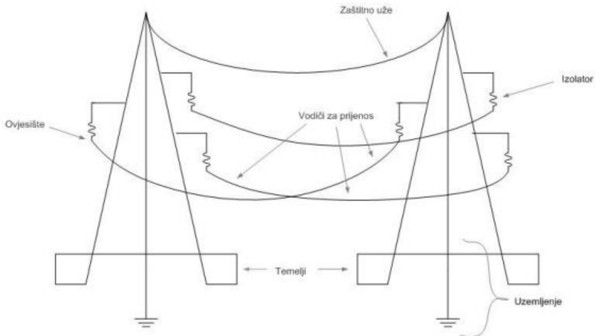
Slika 3.2. Prikaz nadzemnog voda i svih sastavnih dijelova. [6]
