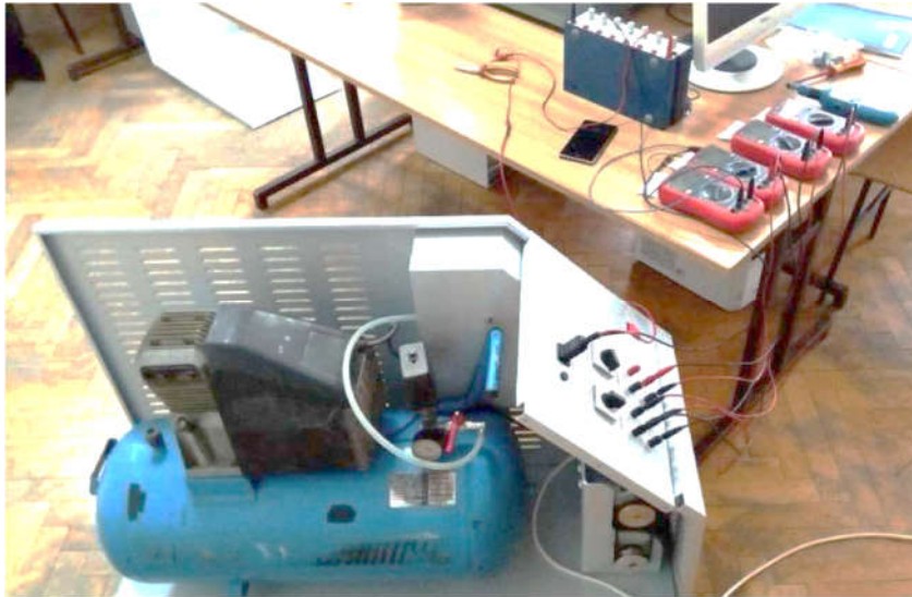
Slika 4.1.: Eksperimentalni postav.
