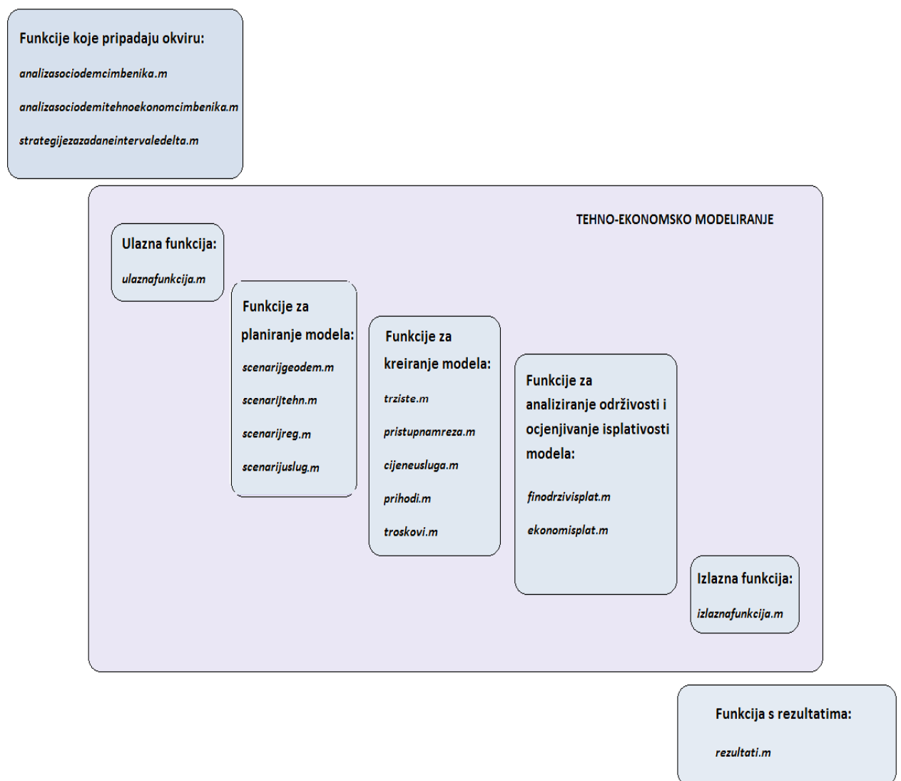
Slika 5.4. Prikaz funkcija u modelu
