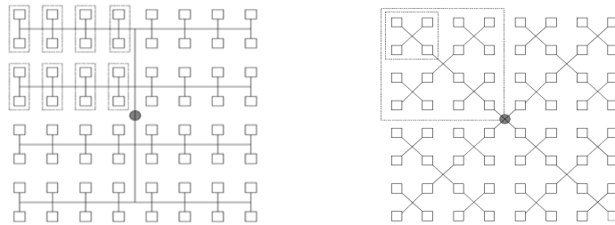
Slika 3.8. Struktura žičnih vodova postavljena duž ulice te dijagonalno [32]
