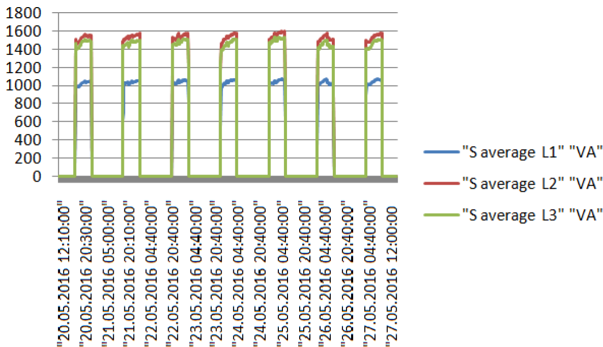
Sl. 4.4. Graf potrošnje prividne snage
