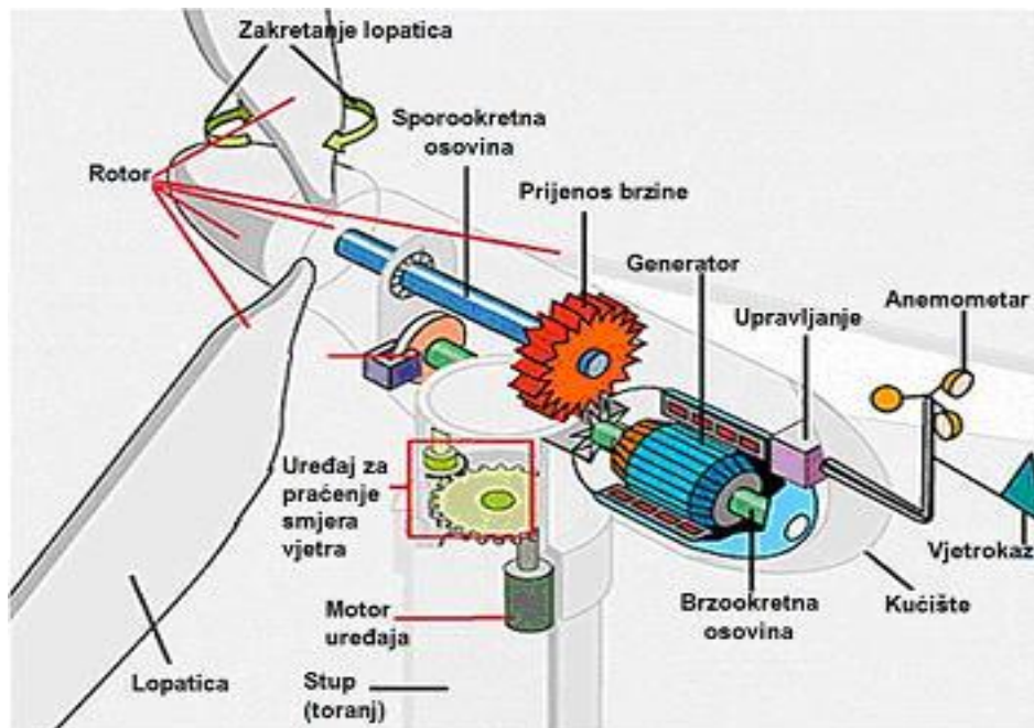
Sl. 3.1. Dijelovi vjetroelektrane [10]
