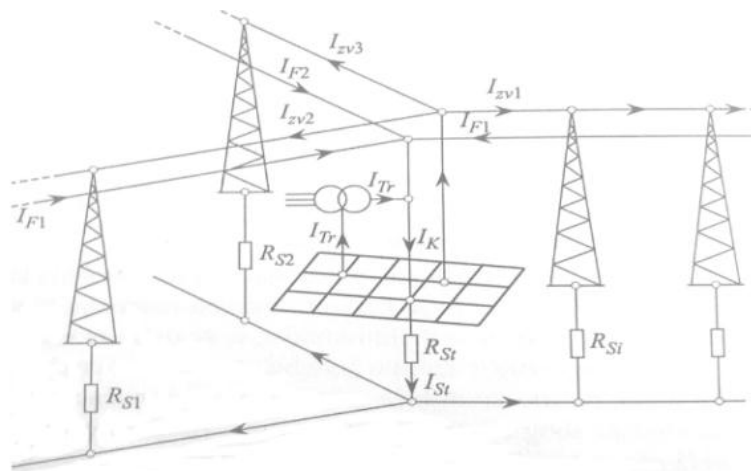
Slika 2.6) Združeno uzemljenje [1]
