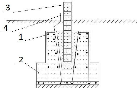
Slika 3.2) temeljna klupa [1]
