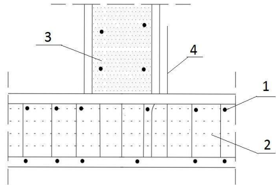
Slika 3.3) temeljna ploča [1]
