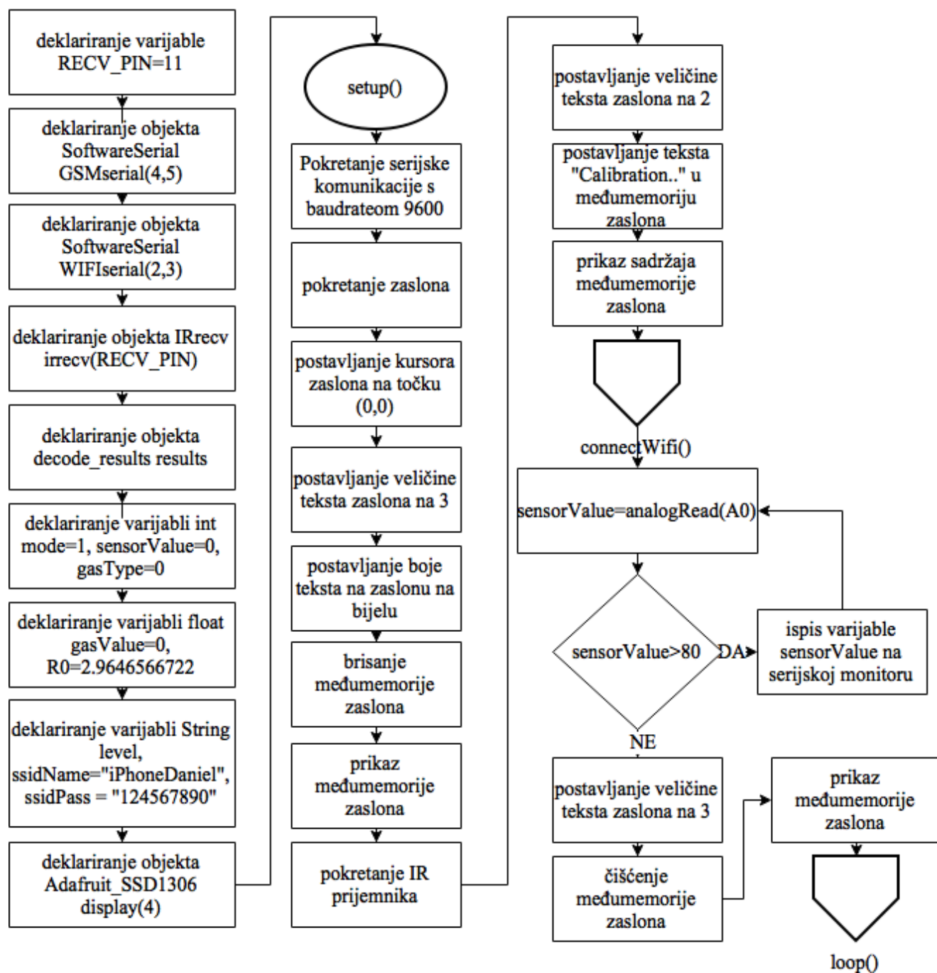
Sl. PE.1. Dijagram toka početka programa i funkcije setup()
