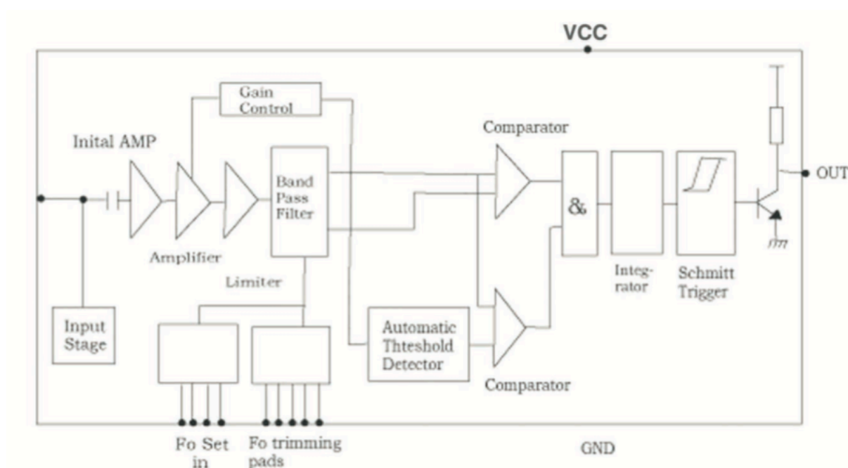
Sl.PC.1. Strujni krug koji opisuje rad IR prijemnika; Izvor: http://datasheetcafe.databank.netdna-cdn.com/wp-content/uploads/2015/11/VS1838B.pdf
