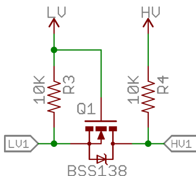
Sl. 2.9. Električna shema pretvornika logičkih razina [13]
