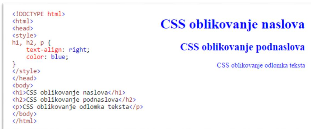
Slika 2.2. Primjer CSS oblikovanja internet stranice: program (lijevo); izgled stranice (desno).
