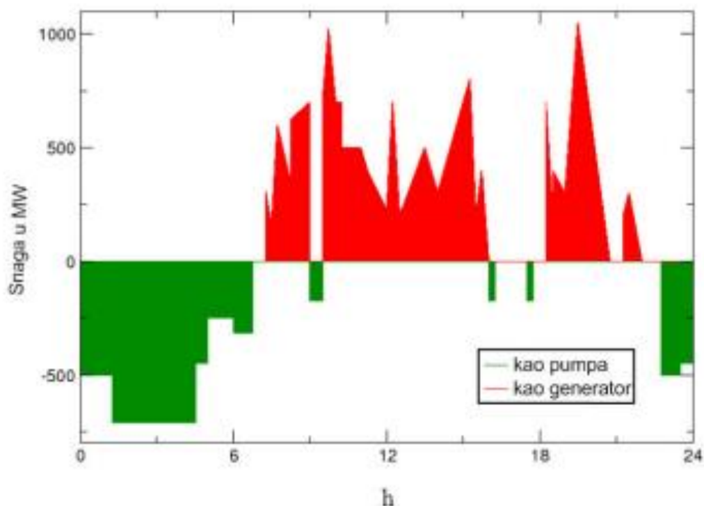
Slika 4.12. Dijagram potrošnje i proizvodnje električne energije
